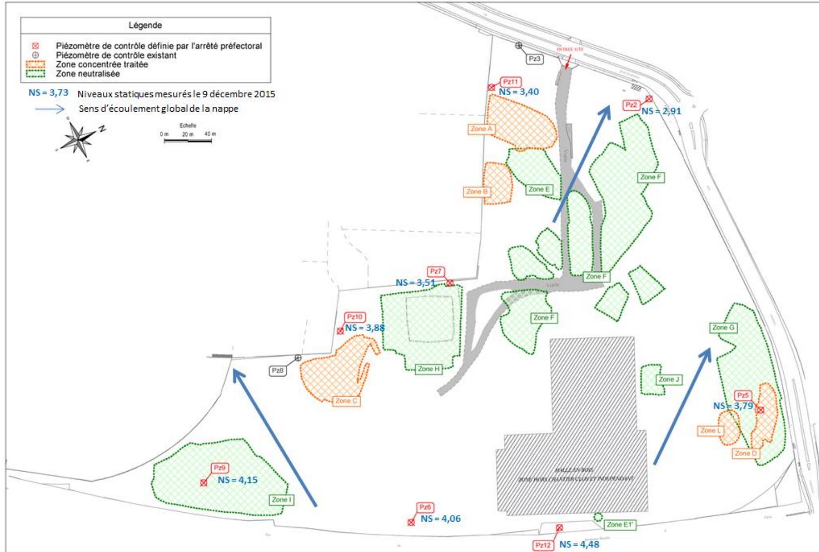
Figure 3 : localisation des piézomètres prélevés dans le cadre de la surveillance (AP 13/11/2013) et des zones traitées – sens d'écoulement global au droit du site et niveaux de la nappe du 9 décembre 2015
